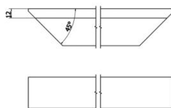
TYP 2 / TYPE 2
