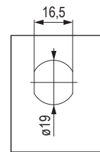
vrtanie otvoru do plechových dverí
