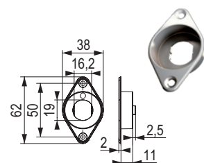
309274 adaptér na montáž do dreva
