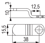
309277 závora 400 zakrivená
