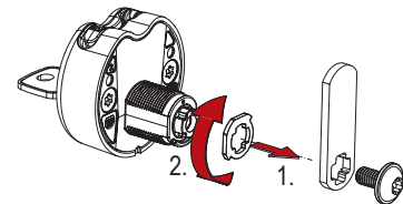
zmena orientácie zámku
