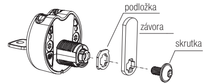
zmena orientácie zámku
