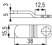
309276 závora 390 zakrivená
