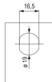
vrtanie otvoru
