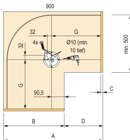
montáž nosnej tyče, korpus 900 mm
