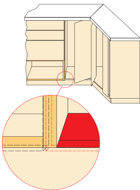
plochu dna zarovnať s hornou hranou sokla
