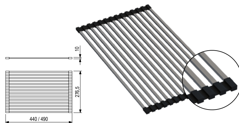
491387 | Rolovací rošt 490 × 277 mm 491388 | Rolovací rošt 440 × 277 mm
