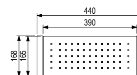
487892 | Odkvapkávacia miska nerez/plastu, pre drezy 482139, 482140, 482141, 482144
