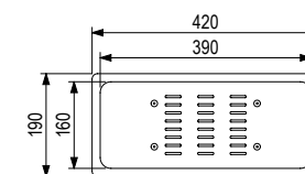
487891 | Odkvapkávacia miska nerez, pre drezy 482141, 482142, 482143, 482144
