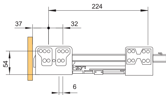
vrtanie otvorov pre dĺžky 270 mm a 300 mm
