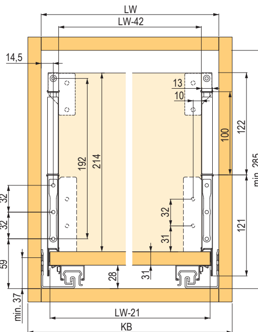
StrongMax zvýšená bočnica 121 mm
