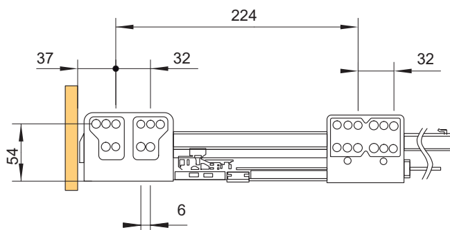
vrtanie otvorov pre dĺžky 350 mm až 550 mm
