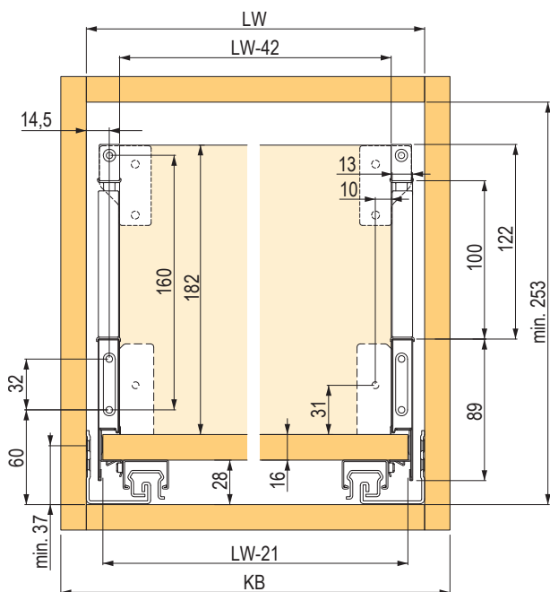
StrongMax zvýšená bočnica 89 mm
