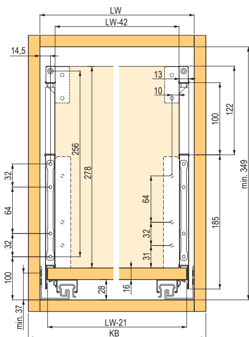
StrongMax zvýšená bočnica 185 mm
