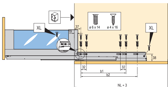
Inlay bočnice z individuálneho materiálu
