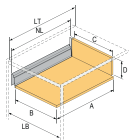
Čelná zásuvka, výška 70/176 mm
