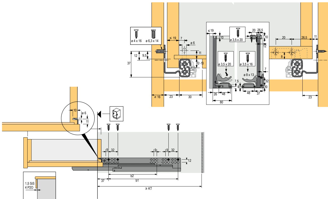
Celovýsuv Quadro V6
