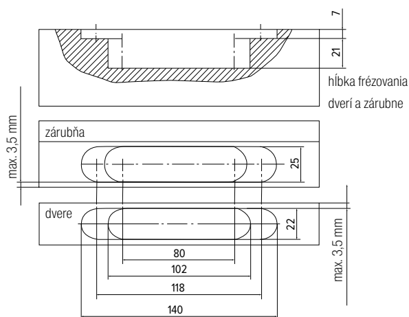
frézovanie dverí a zárubní pre záves Symbio 22
