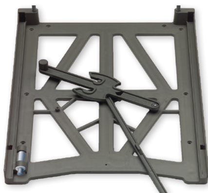
mechanizmus na automatické vysúvanie koša
