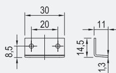
Úhelníková zarážka 30 mm
