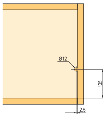
zadný pohľad – otvor na lanko
