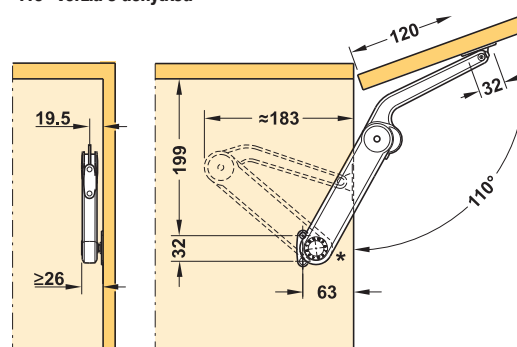
110° verzia s úchytkou
