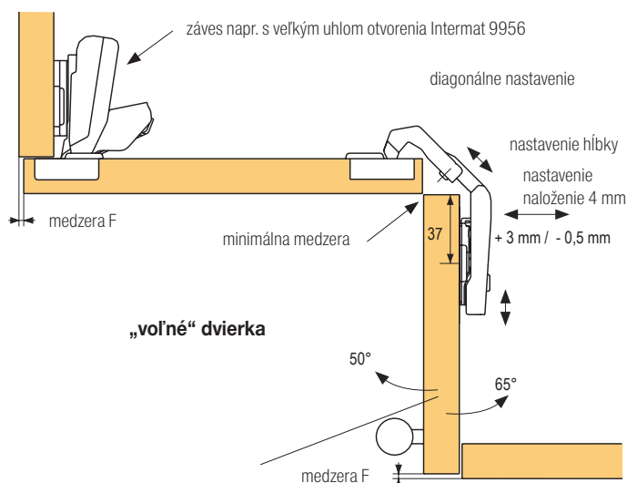
Nákres Variant B
