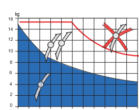
výkonnosť pre dolné vyklápanie 90°
