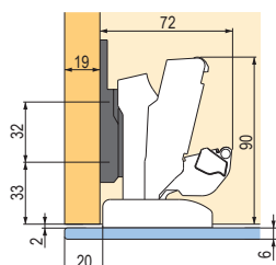
Úplne naložené dvere (bez medzery)
