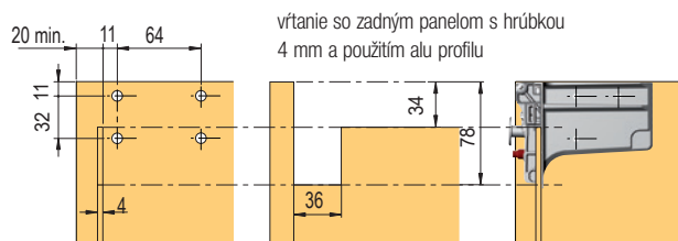
vŕtanie so zadným panelom s hrúbkou 4 mm
