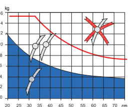
výkonnosť pre horné vyklápanie 90°
