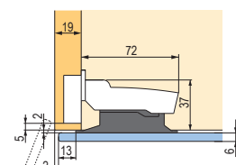
Naložené dvere s medzerou 2 mm
