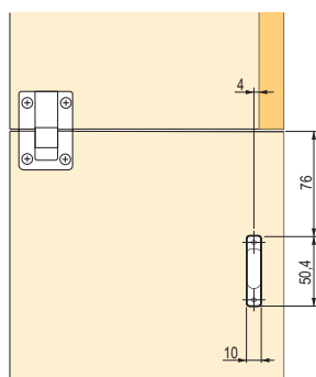
pôdorys – otvor na úchyt dveriek
