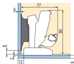
Úplne naložené dvere (bez medzery)
