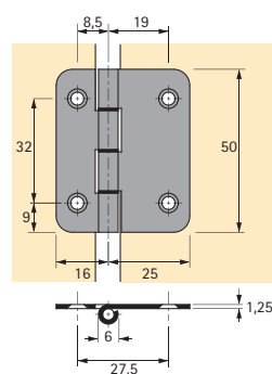
záves 625 pre skladacie dverka
