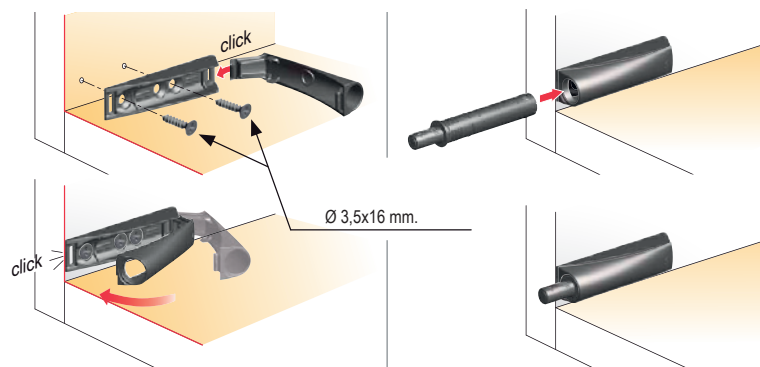
Súprava s adaptérom
