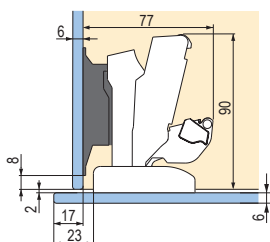
Naložené dvere s presahom dverí 11 mm
