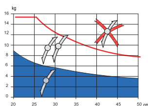
výkonnosť pre horné vyklápanie 75°
