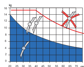
výkonnosť pre horné vyklápanie 75°
