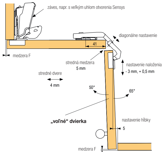
Nákres Variant B
