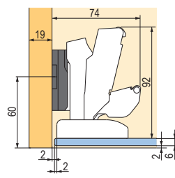
Vložené dvere s odsadením 2 mm
