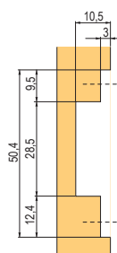
hĺbka zafrézovania otvoru pre úchyt dveriek
