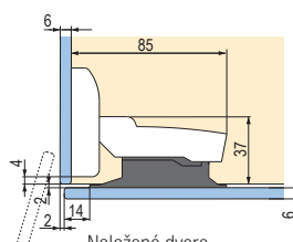
Naložené dvere s medzerou 2 mm
