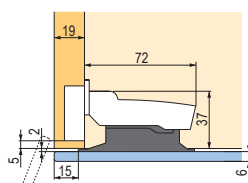
Úplne naložené dvere (bez medzery)
