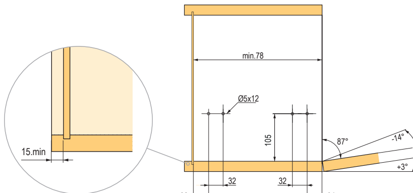
bok korpusu – otvory pre vodiacu lištu
