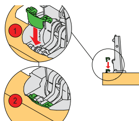
Montáž INSERTA / nalisováním / exp.
