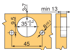
Montáž INSERTA / nalisováním / exp.
