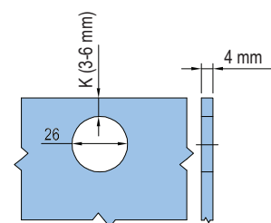
priemer vŕtania
