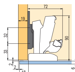
Naložené dvere s medzerou 2 mm
