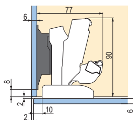
Naložené dvere s medzerou 2 mm
