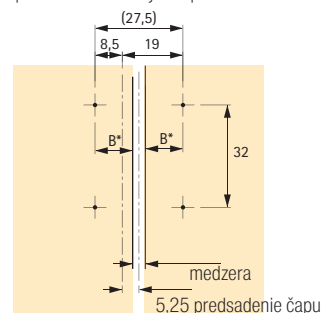
použitie s odsadeným čapom
