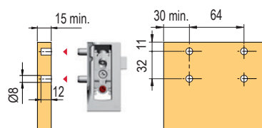
vŕtanie bez zadného panelu
