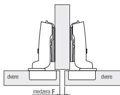
Minimálna medzera (F) medzi jednotlivými dverami (9944)
