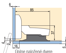
Úplne naložené dvere (bez medzery)
