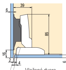
Vložené dvere s medzerou 2 mm
