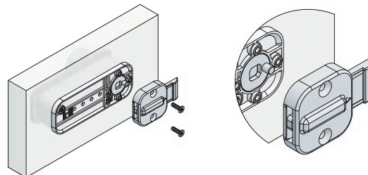
Bolt right locking Riegel rechts
