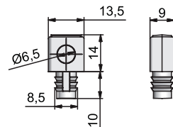
Rod guide with dowels 071 Stangenführung dübelbar 071
