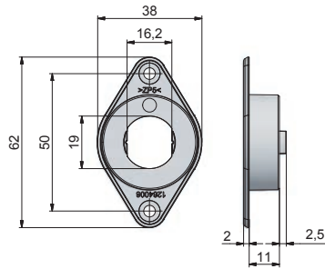
Fixing element 1619 Befestigungsadapter 1619
