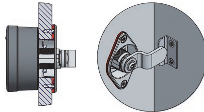
Examples of installation situations Beispiele für Einbausituationen
