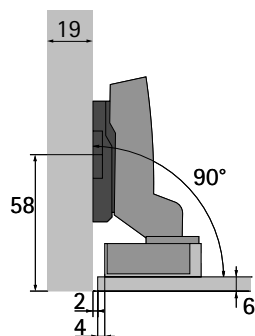
Sensys 8645i B-4 / 8631i B-4 S adaptérem k nalepení pro vložené dveře montážní podložka* distance = 3 mm
