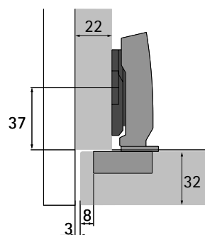
Sensys 8631i B12,5 Silné dveře pro naložené dveře montážní podložka* distance = 1,5 mm
