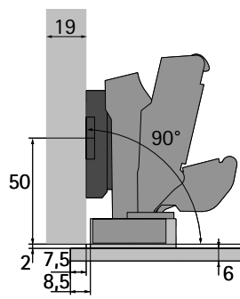
Sensys 8657i B3 S adaptérem k nalepení pro polonaložené dveře montážní podložka* distance = 5 mm omezovač úhlu otevření 120°
