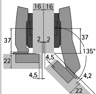
Sensys 8639i W45 B-2 pro naložené dveře montážní podložka* distance = 3 mm
