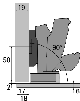
Sensys 8657i B3 S adaptérem k nalepení pro naložené dveře montážní podložka* distance = 5 mm omezovač úhlu otevření 120°
