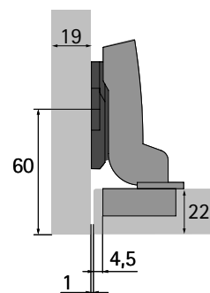
Sensys 8631i B-4 Silné dveře pro vložené dveře montážní podložka* distance = 1,5 mm
