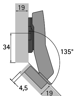
Sensys 8639i W45 B-2 pro naložené dveře montážní podložka* distance = 1,5 mm
