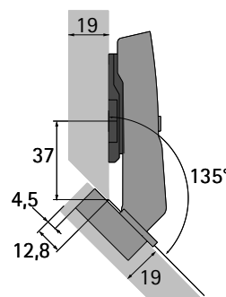
Sensys 8639i W45 B9 pro naložené dveře montážní podložka* distance = 0 mm
