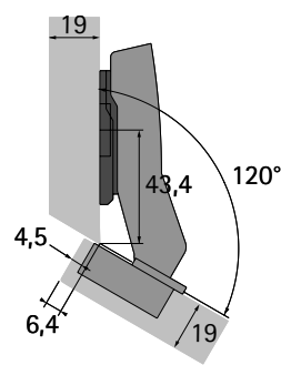
Sensys 8639i W30 B2 pro naložené dveře montážní podložka* distance = 0 mm
