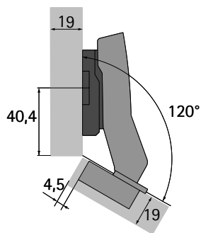
Sensys 8639i W30 B2 pro naložené dveře montážní podložka* distance = 5 mm
