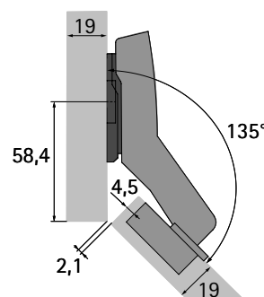
Sensys 8639i W45 B-25 pro vložené dveře montážní podložka* distance = 0 mm
