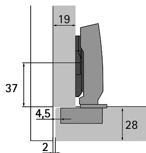
Sensys 8631i B12,5 Silné dveře pro naložené dveře montážní podložka* distance = 0 mm
