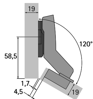
Sensys 8639i W30 B-16 pro vložené dveře montážní podložka* distance = 1,5 mm
