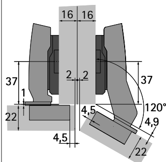
Sensys 8639i W30 B2 pro naložené dveře montážní podložka* distance = 3 mm
