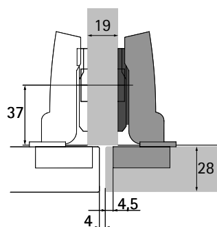
Sensys 8631i B3 Silné dveře pro polonaložené dveře montážní podložka* distance = 0 mm
