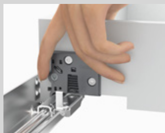
Seřízení sklonu
