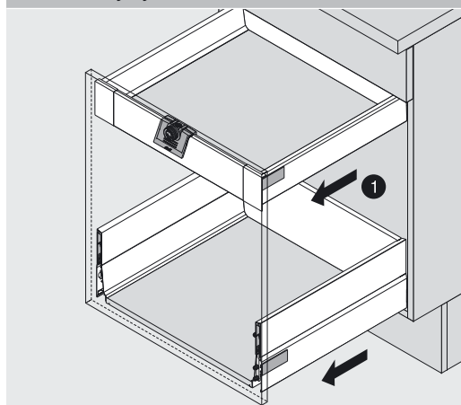
Aktivace unašeče
