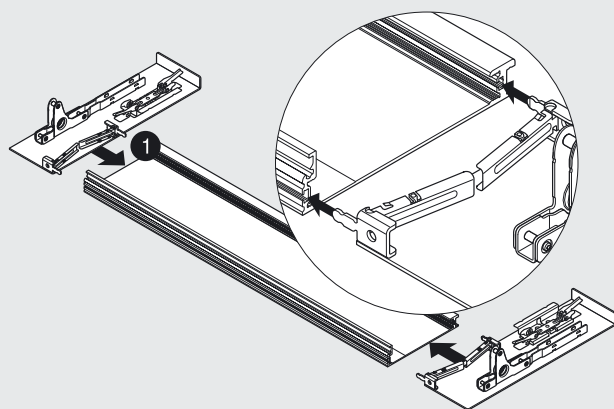
Montáž předního dílu
