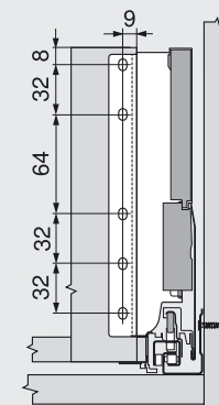
Montážní míry pro záda
