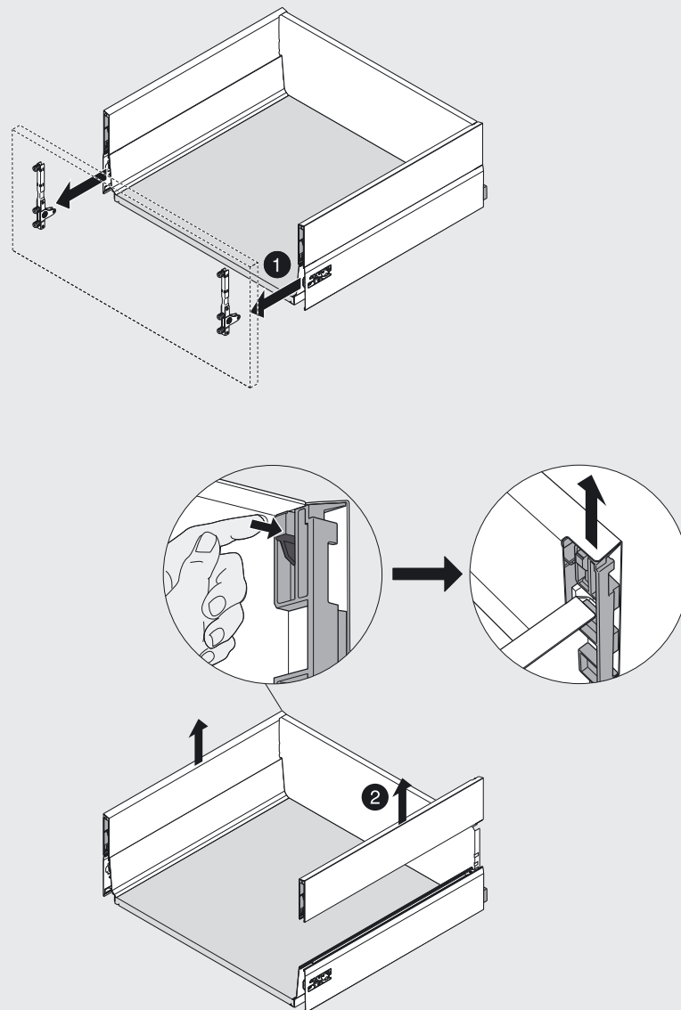
Demontáž BOXCAP
