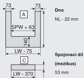
Rozměry přířezů pro dřevotřísku 16 mm
