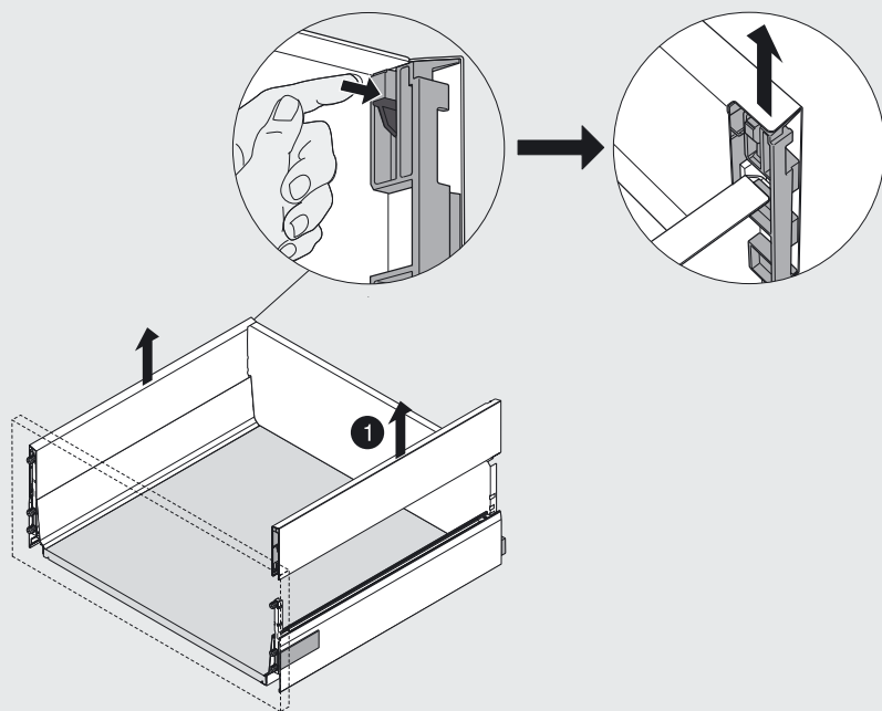
Demontáž BOXCAP
