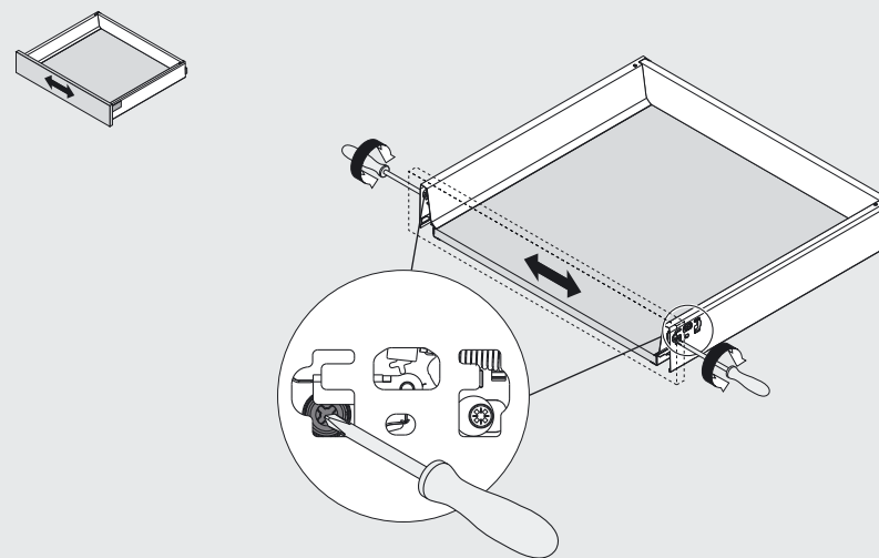
Boční nastavení
