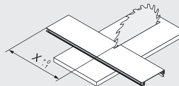
Zkrácení předního dílu s drážkou
