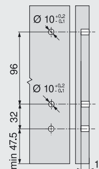
Rozměry pro vyvrtání otvorů u čela pro EXPANDO
