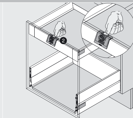
Odblokování
