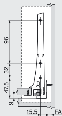
Konstrukční rozměry pro montáž čela vruty
