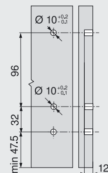
Rozměry pro vyvrtání otvorů u čela pro EXPANDO
