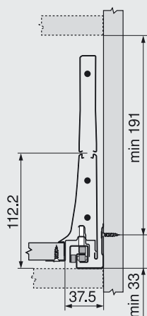
Potřebný prostor v korpusu
