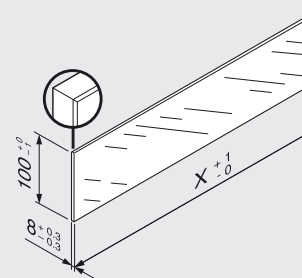
Rozměry přířezů zásuvného prvku
