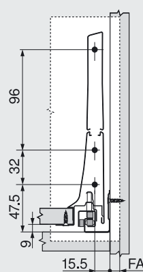
Konstrukční rozměry pro montáž čela vruty
