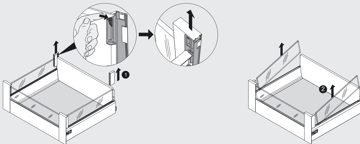
Demontáž zásuvného prvku
