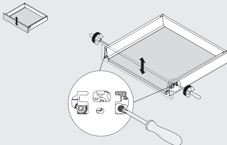
Nastavení výšky
