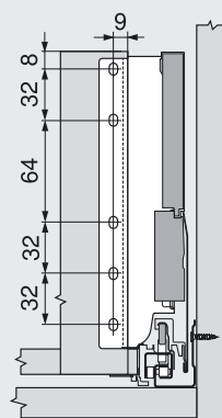
Montážní míry pro záda
