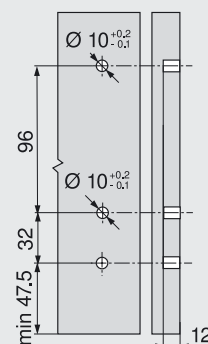
Rozměry pro vyvrtání otvorů u čela pro EXPANDO
