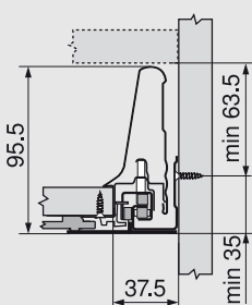
FA Presah čela
