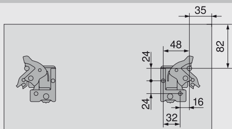
Dno zásuvky voľné, Ø 5 mm
