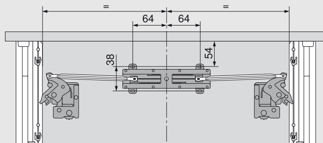
Dno zásuvky 3-stranné predmontované, Ø 5 mm
