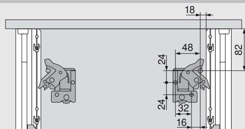
Dno zásuvky 3-stranné predmontované, Ø 5 mm
