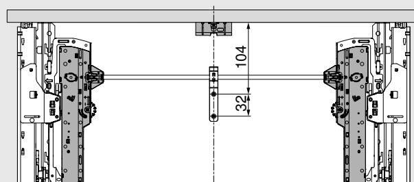
TIP-ON BLUMOTION jednotka L1, L3, L5 (NL \geq 350 –650 mm)
