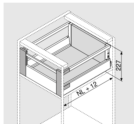
Vnútorý výsuv – výška D
