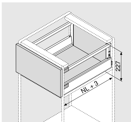
Vnútorý výsuv – výška C
