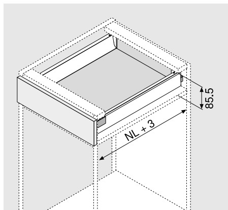
Čelný výsuv – výška C
