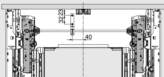
TIP-ON BLUMOTION jednotka L1, L3, L5 (NL \geq 350 –650 mm)
