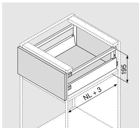
Vnútorá zásuvka – výška K
