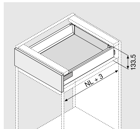
Vnútorá zásuvka – výška M
