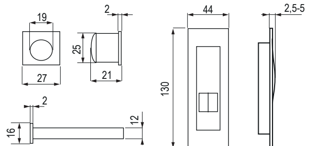
frézovací otvor hĺbka 11 mm
