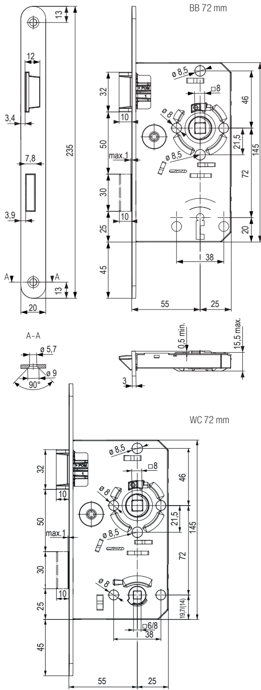
plastová strelka závora BB/72 mm
