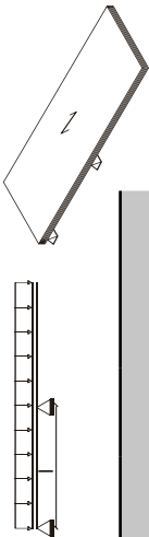
Nosník o jednom poli s konzolou: Zatížení kolmo k rovině desky a paralelně ke směru vláken povrchové vrstvy
